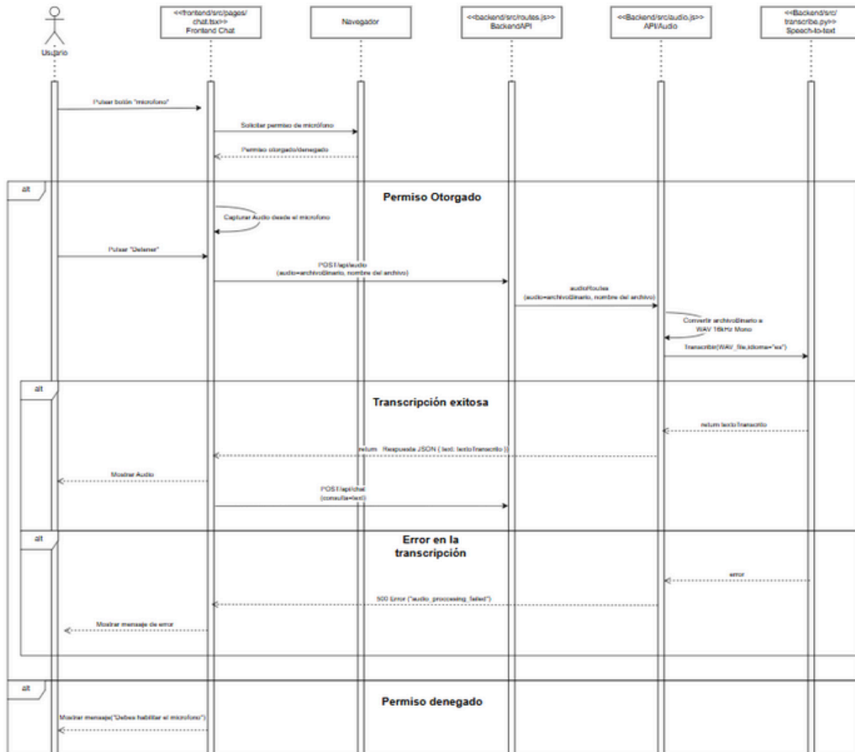
Figura 6. Diagrama de secuencia hacer consulta por audio original ValdivIA
