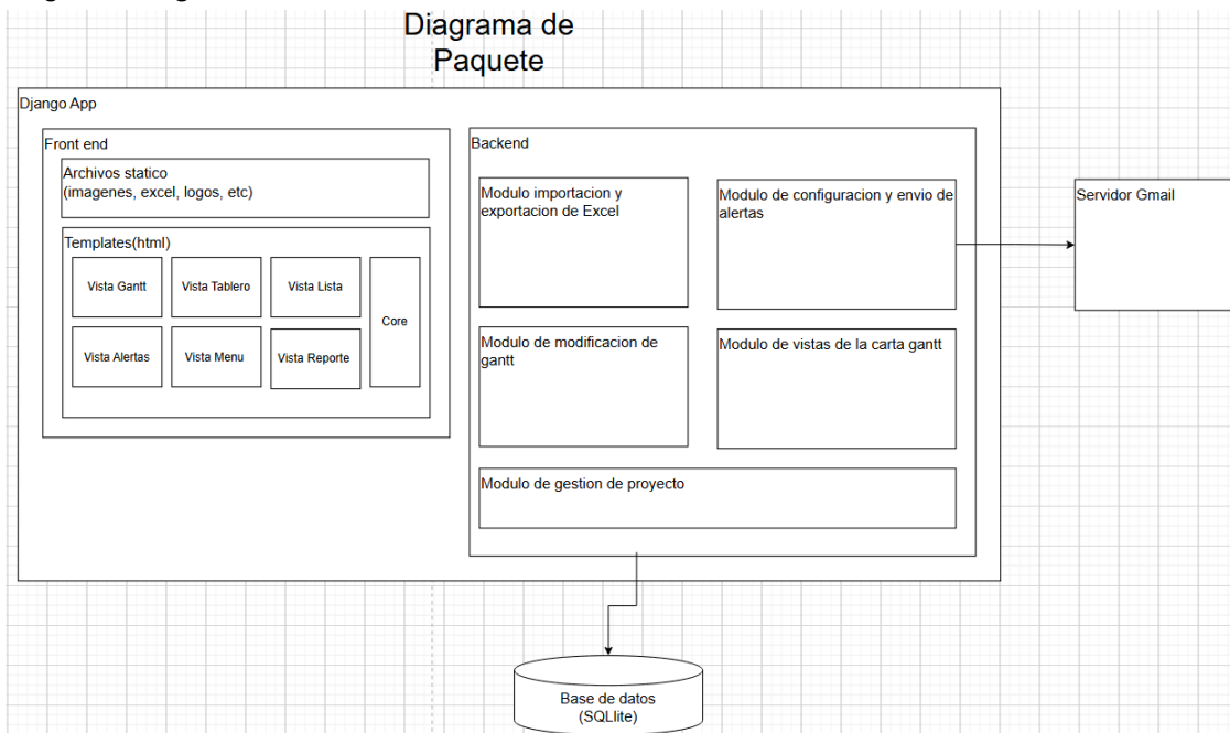
Figura 1. Diagrama de Paquete
