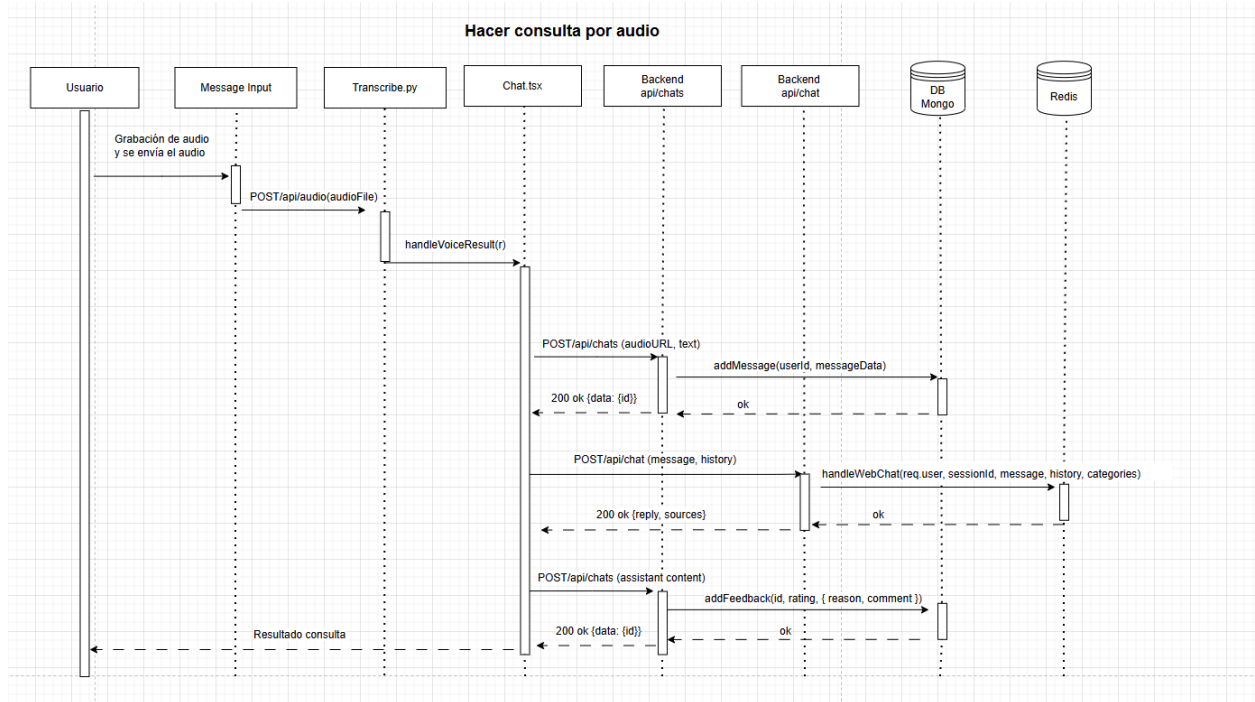
Figura 3. Diagrama de secuencia hacer consulta por audio
