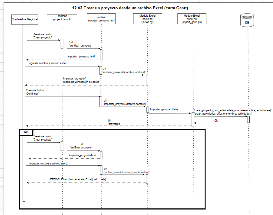
Figura 2. Diagrama de secuencia H2
