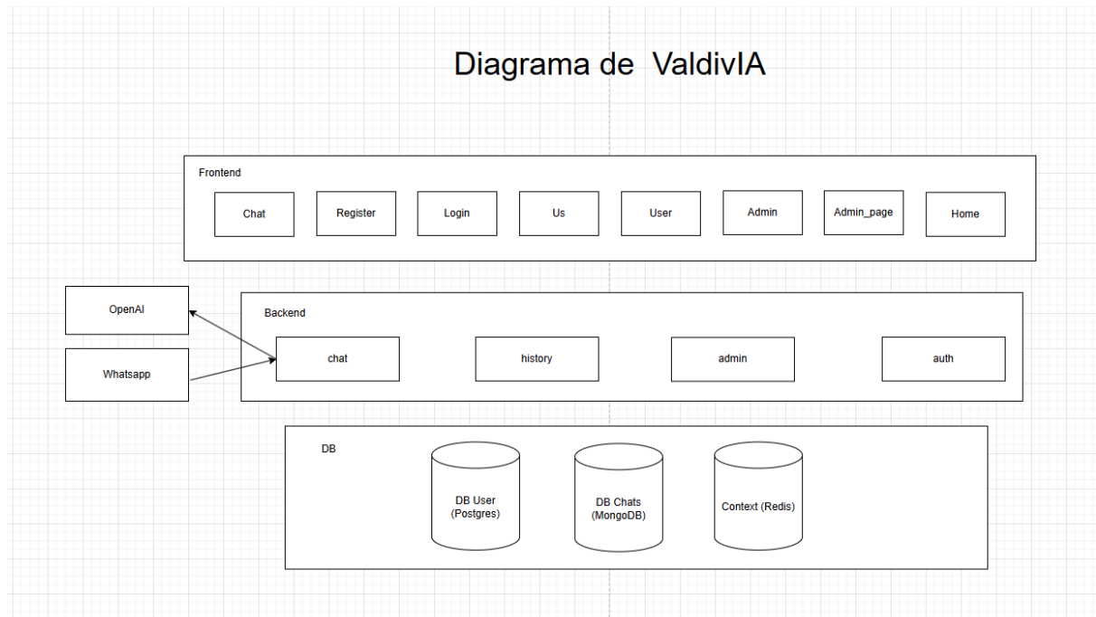
Figura 4. Diagrama de Paquetes ValdivIA
